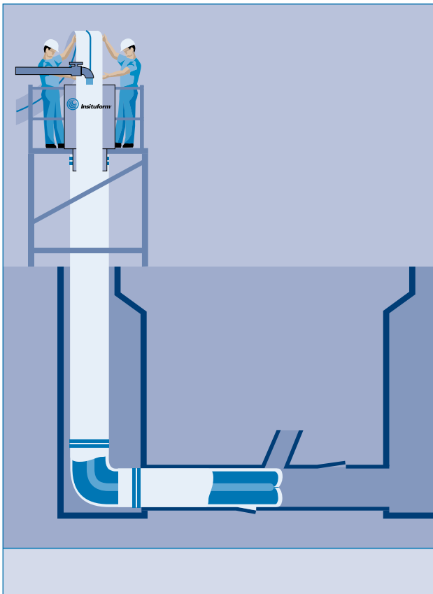
Inversion des Insituform® Schlauchliners
