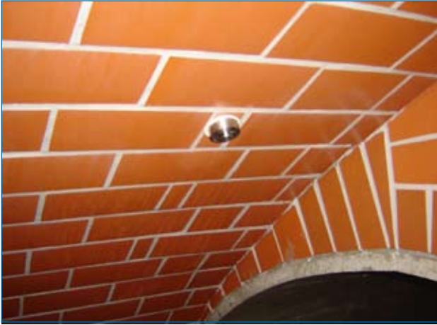
Mit Kera-Line-Platten ausgekleidetes Bauwerk
