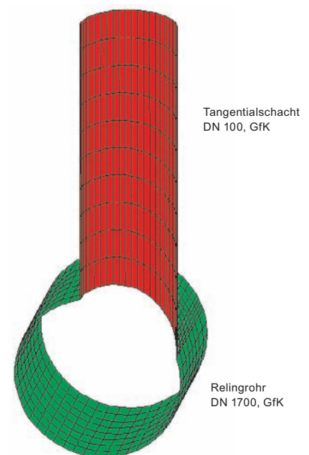
Bild 4: Beispiel eines räumlichen FE-Modells für die Anbindung eines Tangentialschachtes an einen zuvor eingebauten GfK-Inliner Fig. 4: Example of a 3D FEM model for connection of a tangential shaft to a previously installed GRP Inliner
