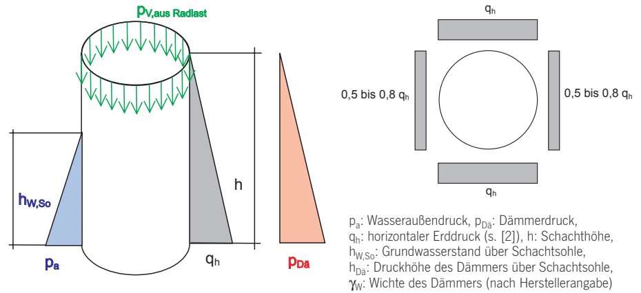
Bild 3: Lastansätze für die Schachtsanierungen: links) Räumliche Darstellung; rechts) Lastansätze für die Schachtsanierungen (Horizontalschnitt, Einwirkung von Erd- und Verkehrslasten q_h ) Fig. 3: Load assumptions for shaft refurbishing: left) 3D view; right) horizontal section, effects of soil and traffic loads q_h
