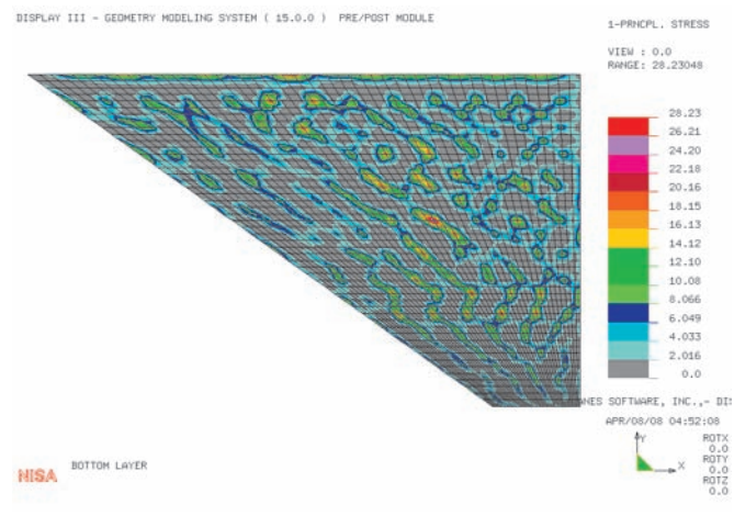
Bild 9: Darstellung der 1. Hauptspannung [N/mm²] in den GfK-Platten unter Einwirkung der Gebrauchslast Fig. 9: View of first principal stress [N/mm²] in the GRP panels under the effects of service load
