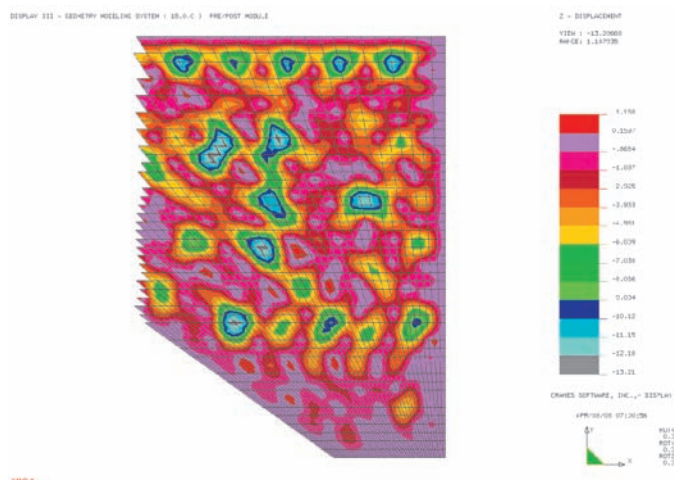
Bild 8: Darstellung der Vertikaldeformationen des ausgekleideten des ausgekleideten Sohlbereiches im Verschneidungsbereich zwischen zwei Großrohren Fig. 8: View of vertical deformations of the lined shaft-bottom zone in the area of intersection of two large-caliber pipes
