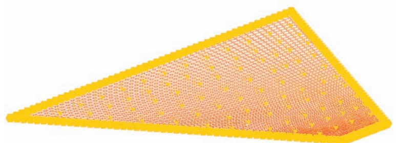
Bild 7: Darstellung des ausgekleideten Sohlbereiches im Verschneidungsbereich zwischen zwei Großrohren Fig. 7: View of the lined shaft-bottom zone in the area of intersection of two large-caliber pipes
